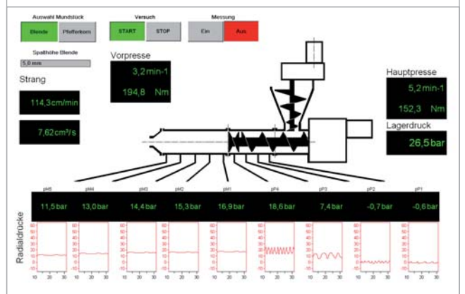
Beispiel eines ESM Versuchsaufbaus
