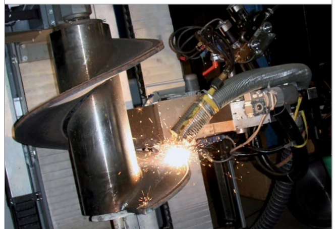
Regenerierung einer Extruderschnecke am Schweißautomat
