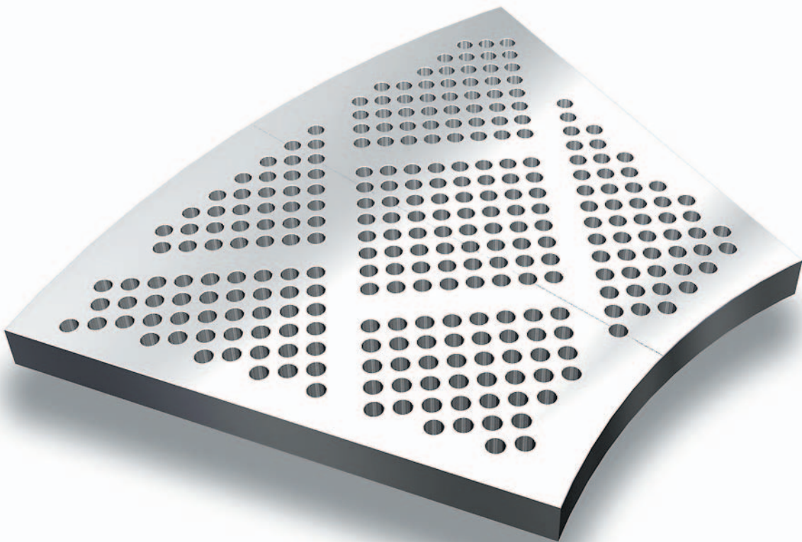
Maßgeschneiderte Konfiguration und Perforation der Rostplatten - auch für Maschinen anderer Fabrikate.
